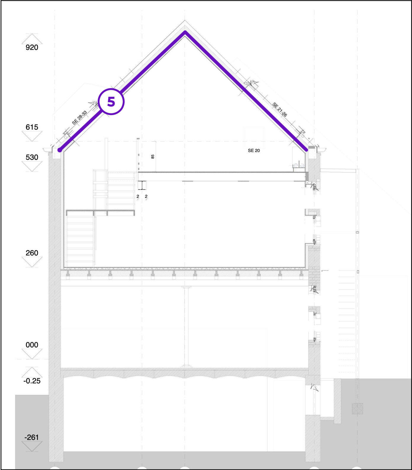
Legende van plan 1.5: Doorsnede kantoren
