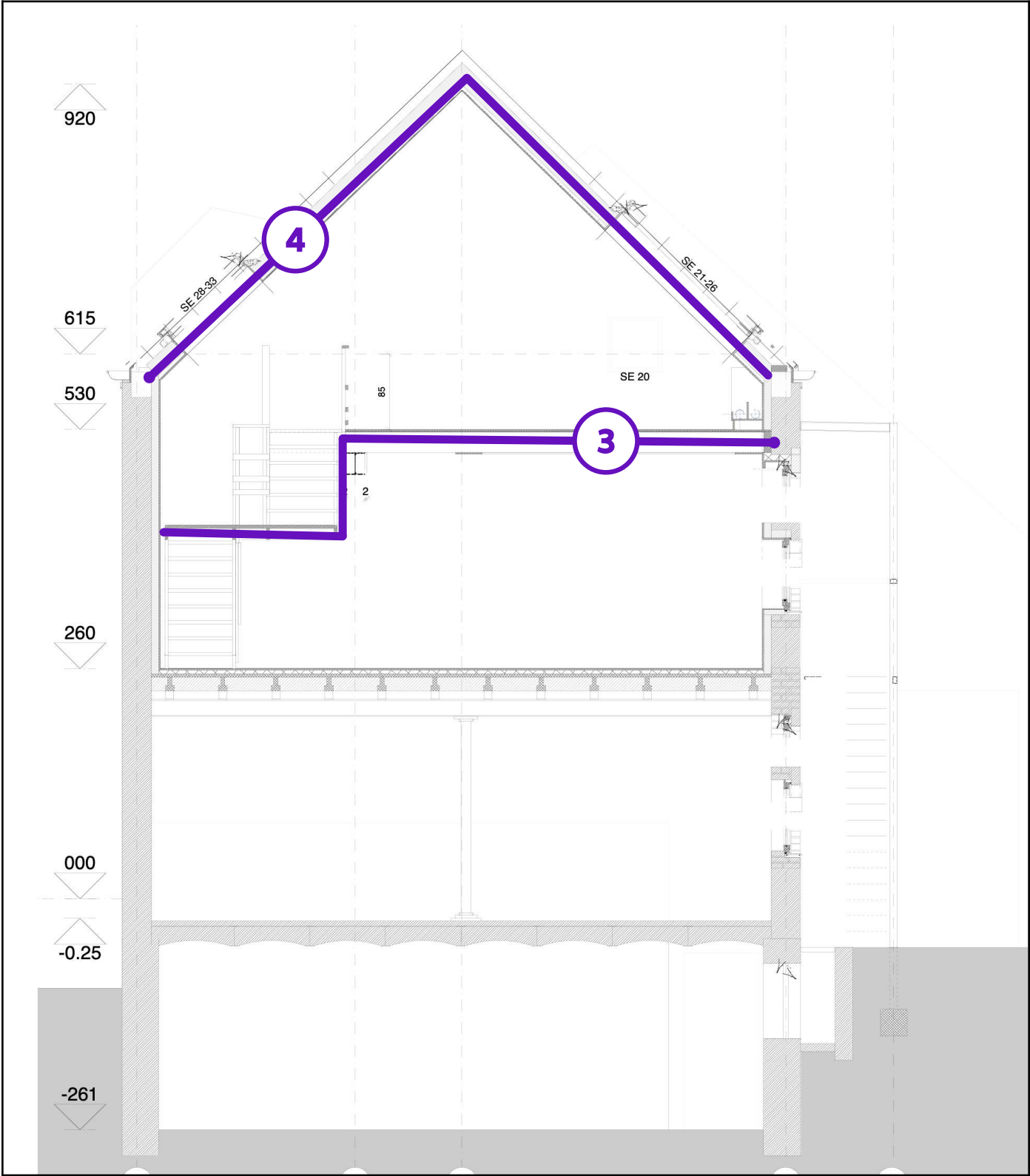
Legende van plan 1.3: Doorsnede kantoren
